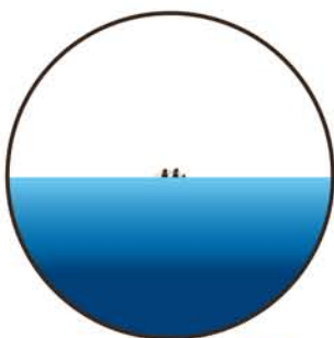
Menschliches Auge
